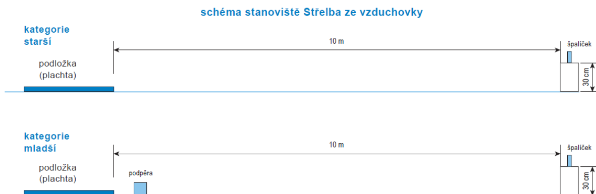
Obr. 1 Střelba – Schéma stanoviště střelba ze vzduchovky
